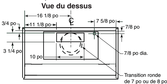
MODÈLE RMIP33 AVEC VENTILATEUR 331H, 332H, 335, 336, HLB3, HLB6, HLB9 OU HLB11 (sortie verticale)
