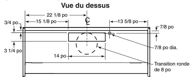
MODÈLE RMIP45 AVEC VENTILATEUR P5 (sortie verticale)
