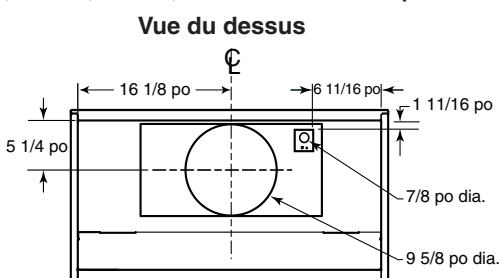
MODÈLE RMIP33 AVEC VENTILATEUR 331H, 332H, 335, 336, HLB3, HLB6, HLB9 OU HLB11 (sortie verticale)
