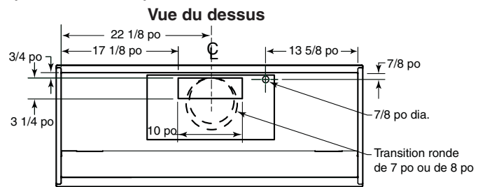
MODÈLE RMIP45 AVEC VENTILATEUR 331H, 332H, 335, 336, HLB3, HLB6, HLB9 OU HLB11 (sortie verticale)
