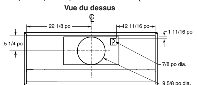
MODÈLE RMIP45 AVEC VENTILATEUR 331H, 332H, 335, 336, HLB3, HLB6, HLB9 OU HLB11 (sortie verticale)
