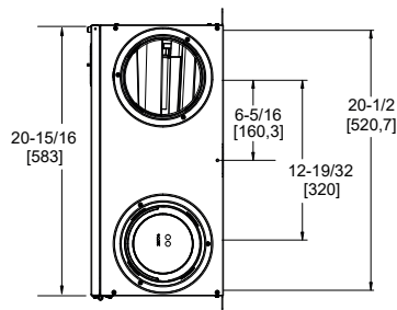
FENTE: Ø3/16 x 1-13/32 [Ø4,8 x 35,6] TROU DU CENTRE: Ø7/16 [Ø11,1]
