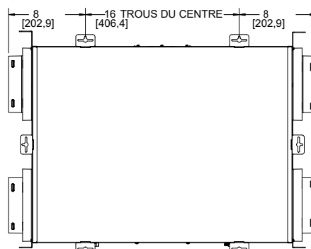
FENTE: Ø3/16 x 1-13/32 [Ø4,8 x 35,6] TROU DU CENTRE: Ø7/16 [Ø11,1]
