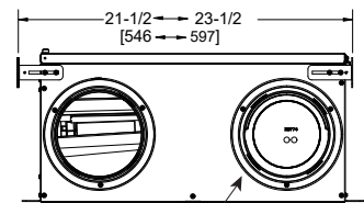
VOLET MOTORISÉ
