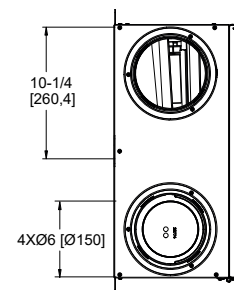
VOLET MOTORISÉ
